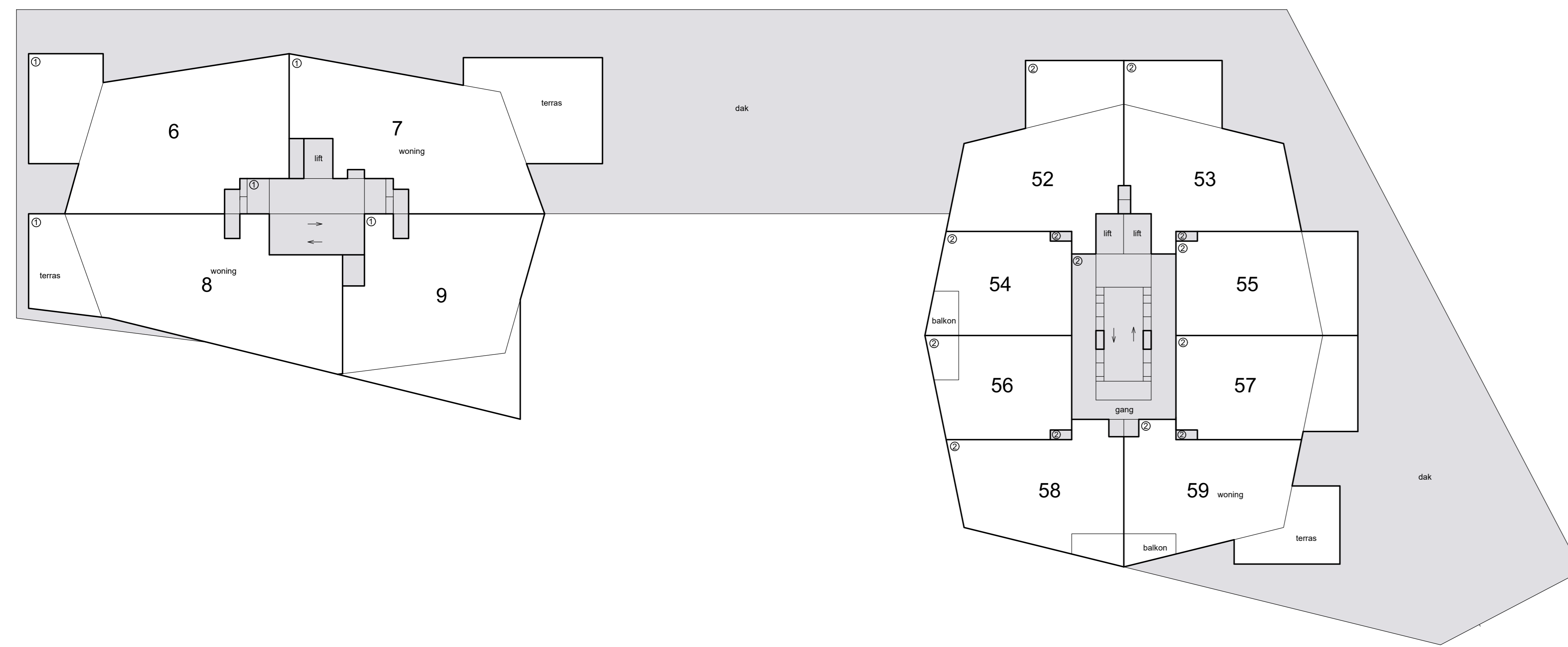
3e etage
